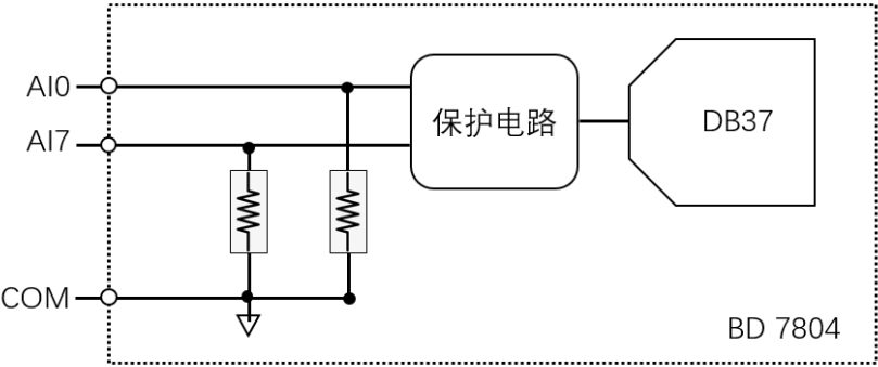
BD 7804 某通道的电路示意图
